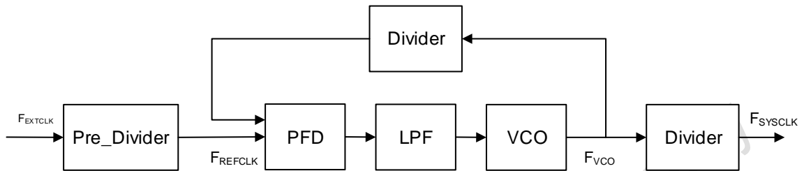
图 1-12 PLL 控制示意图
