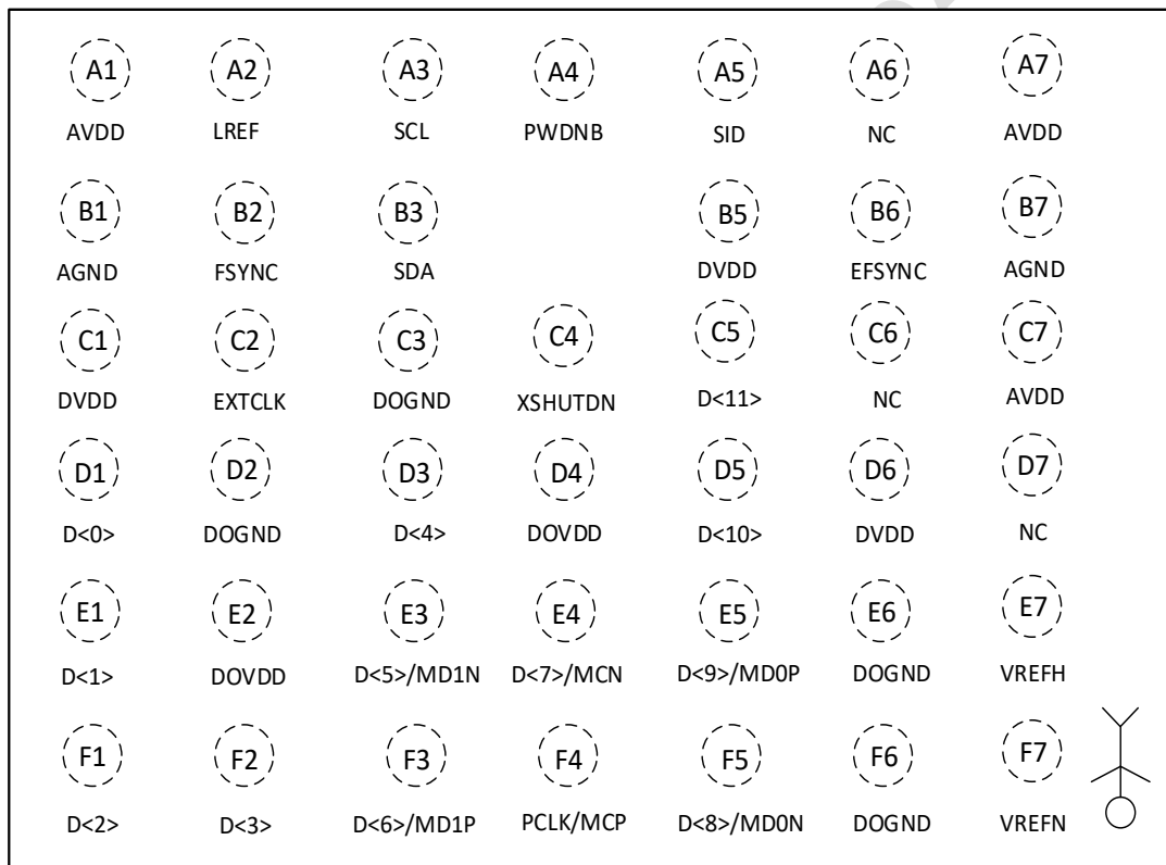
图 1-3 封装引脚图
