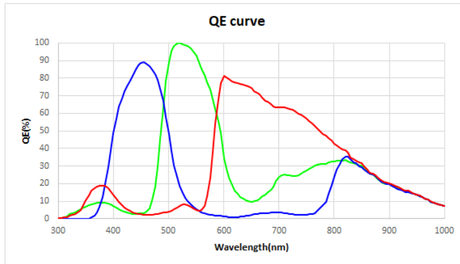
图 4-1 QE 曲线
