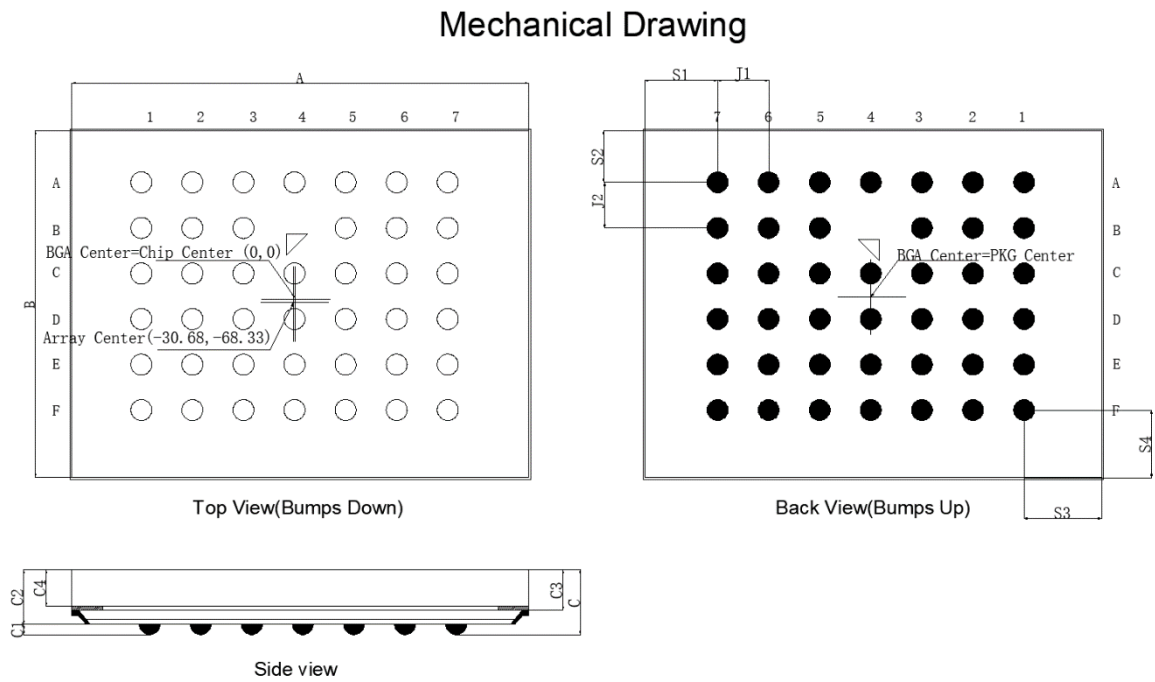
图 5-1 封装示意图
