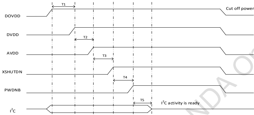
图 1-4 上电时序图
