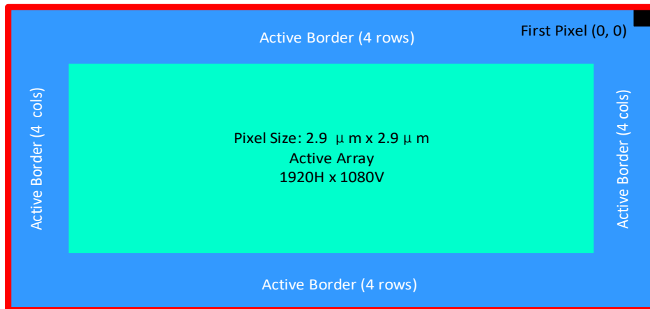
图 2-6 像素阵列图一
